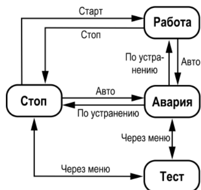
Рисунок 10.1 – Основные режимы работы
