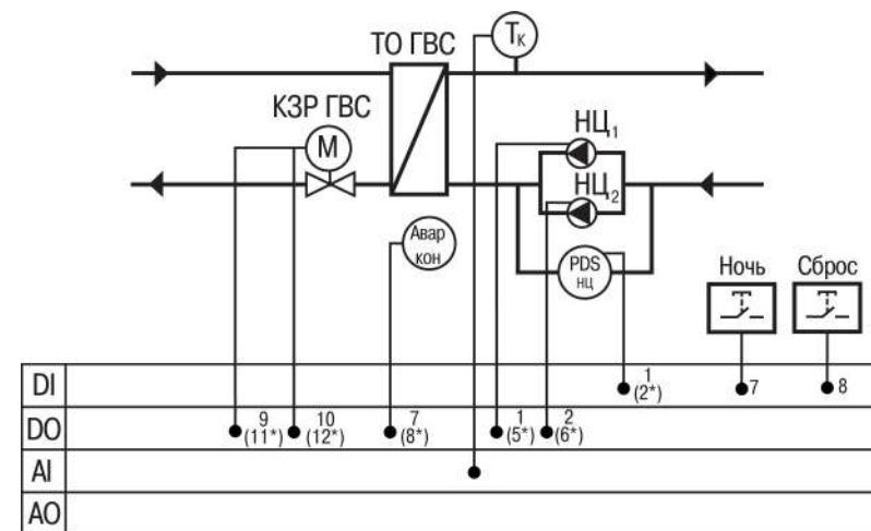
Рисунок 4.2 – Функциональная схема контура «ГВС»
