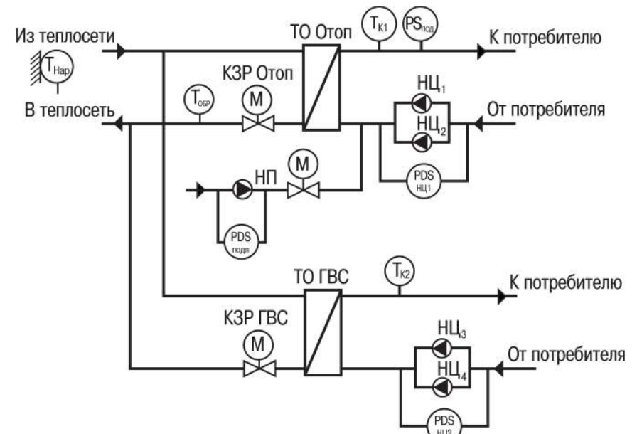
Рисунок 3.3 – Схема контура «Отопление + ГВС»
