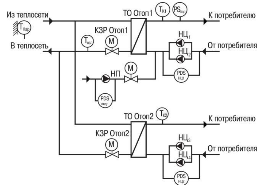
Рисунок 3.4 – Схема контура «Отопление + отопление»
